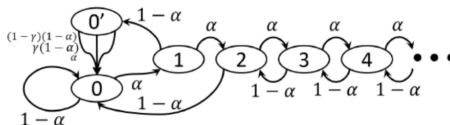
איור 22 - מכונת מצבים המתארת את מצב הבלוקצ'יין של מיינר
