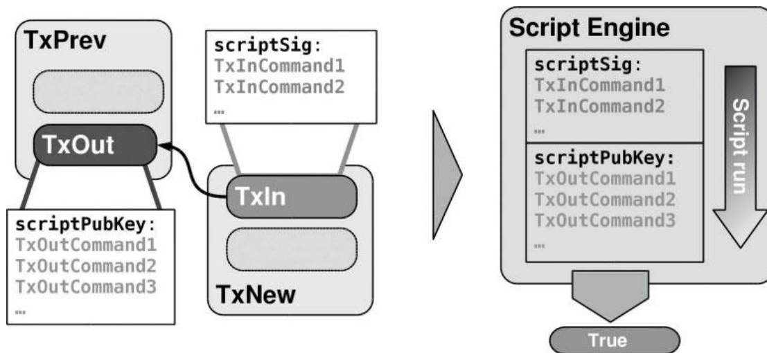
איור 4 - סקריפטי טרנזקציות ומנוע ההרצה
